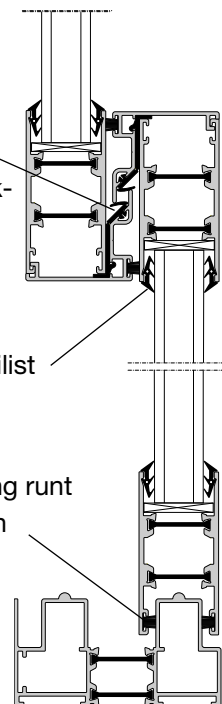
Horisontellt snitt
